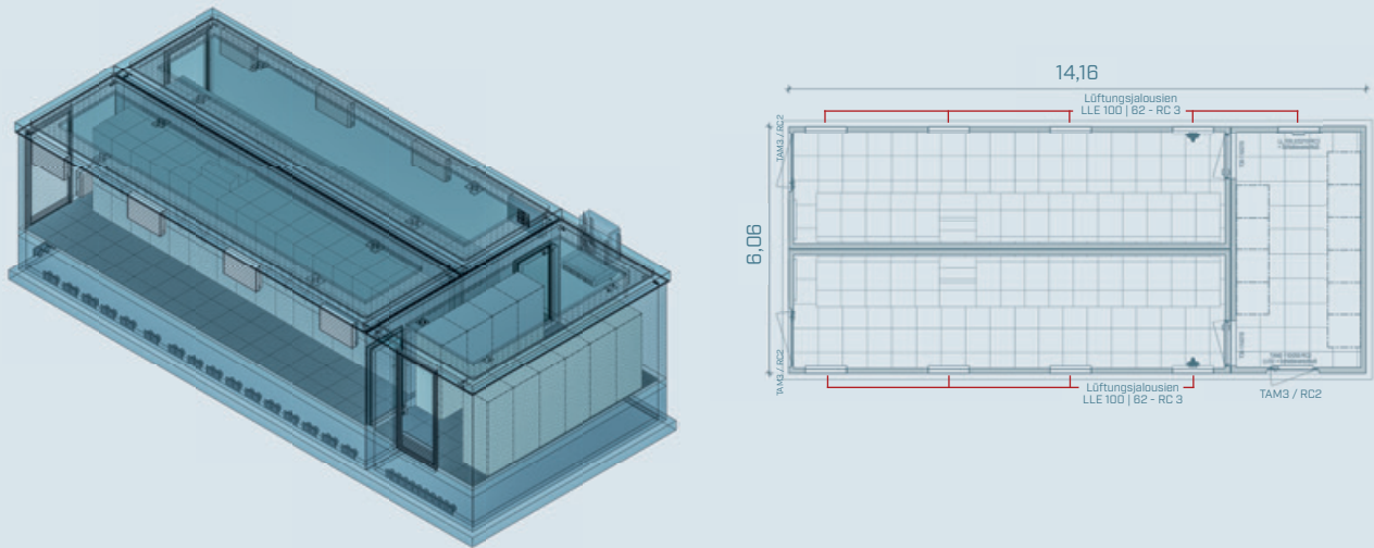
Modularer Aufbau eines Rechenzentrums mit drei Raumzellen
