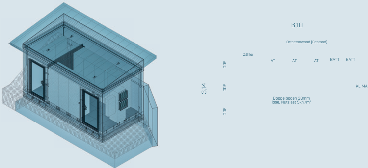
Getrennte Zugänglichkeit von Aktiv- und Passivtechnik durch Gittertrennwand
