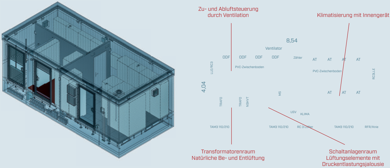
Glasfasertechnik und Energieverteilung unter einem Dach
